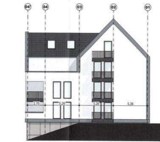
A ONO Ansicht Ost-Nordost 1:200
