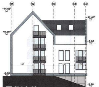
A WSW Ansicht West-Südwest 1:200
