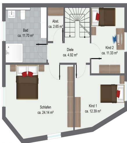
Obergeschoss
