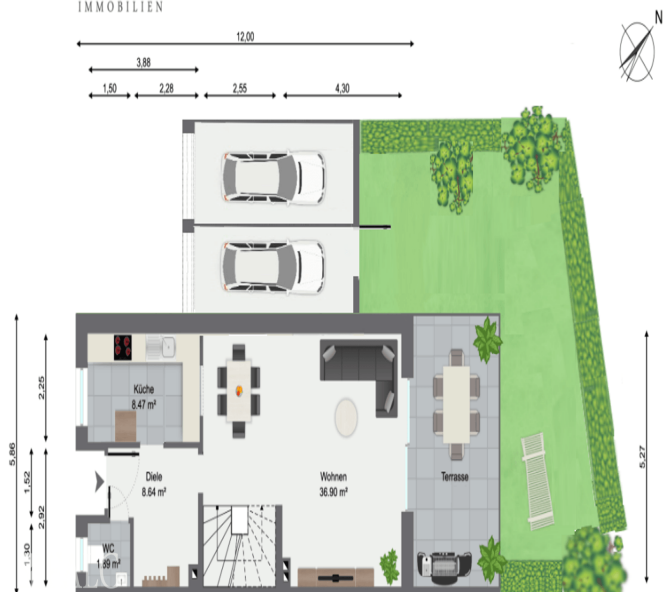
Erdgeschoss
