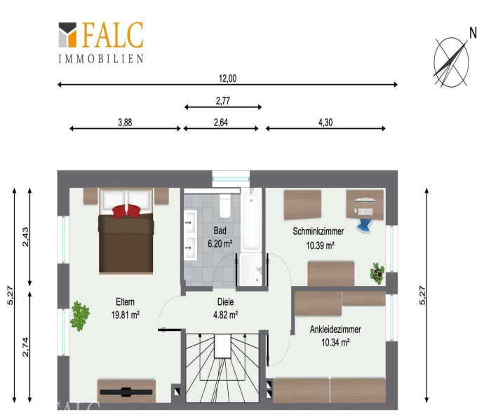
Obergeschoss
