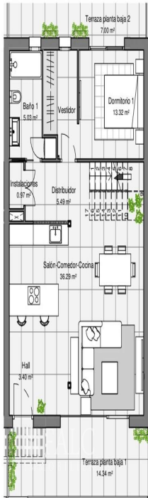
PLANTA BAJA
