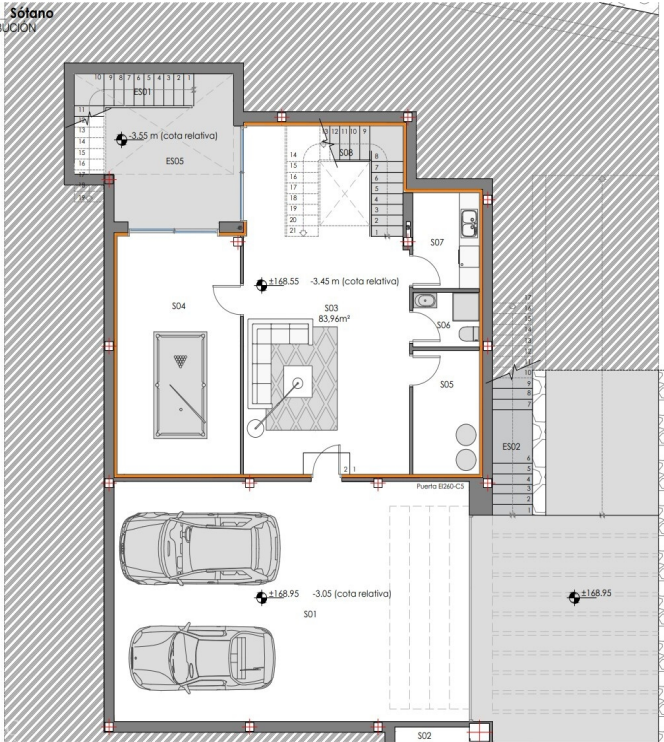
Planta Baja DISTRIBUCIÓN
