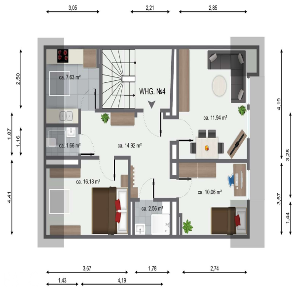
Dachgeschoss
