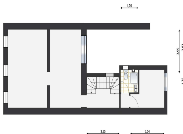
2. Obergeschoss
