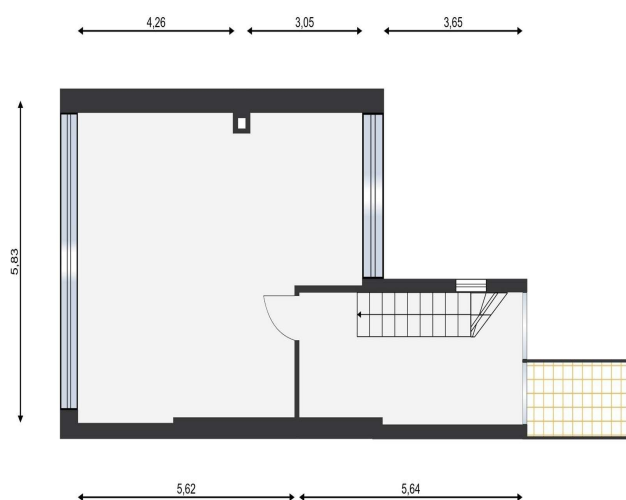
Dachgeschoss
