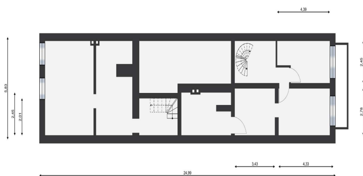
Kellergeschoss
