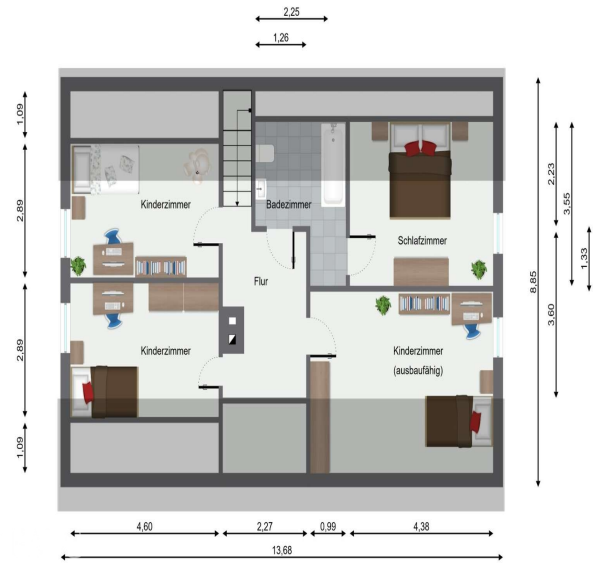
Dachgeschoss
