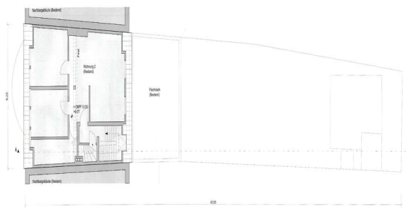
Grundriss Dachgeschoss
