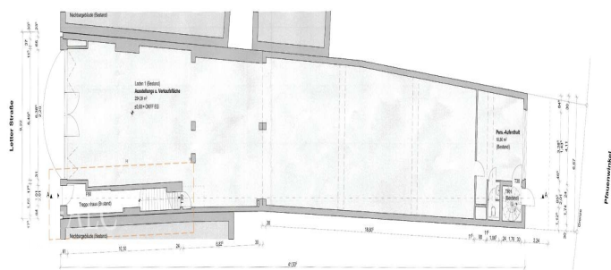
Grundriss Erdgeschoss
