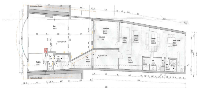
Grundriss 1. Obergeschoss
