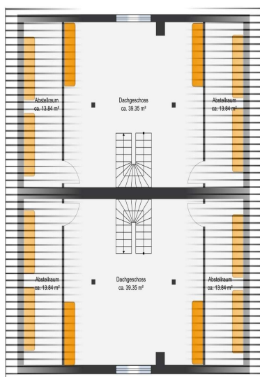
Dachgeschoss
