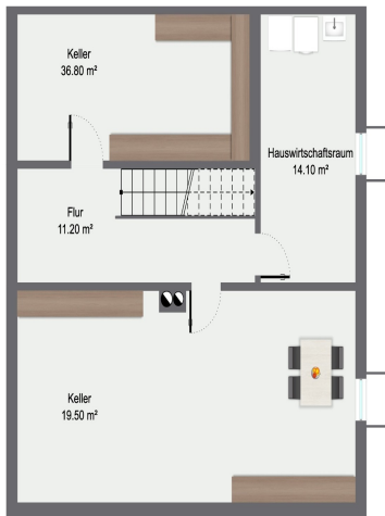
Kellergeschoss
