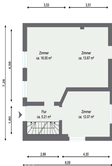
Erdgeschoss
