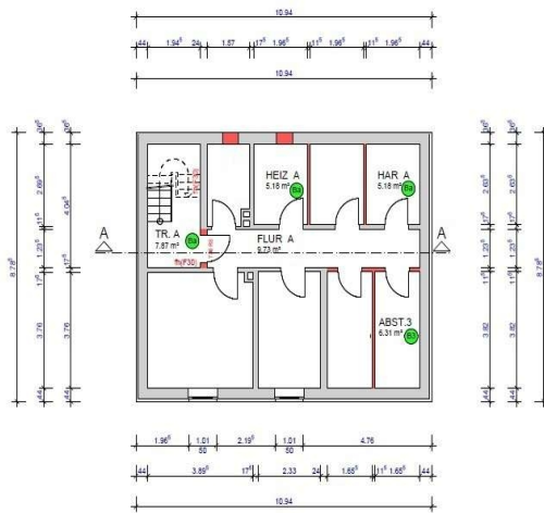
Kellergeschoss
