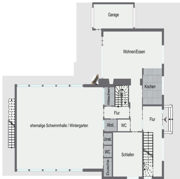
Erdgeschoss
