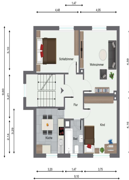
1. Obergeschoss
