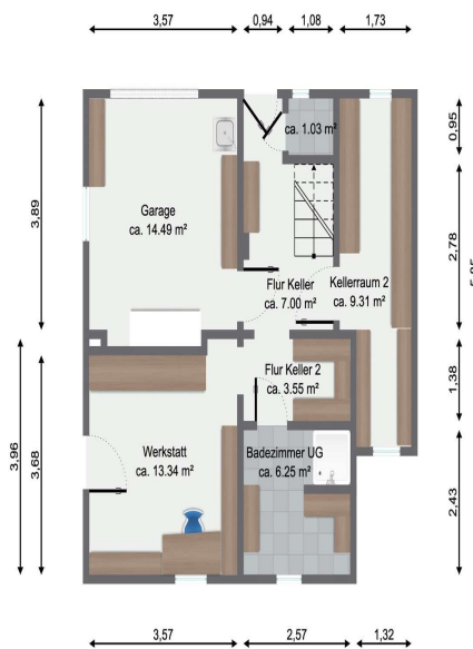
Untergeschoss
